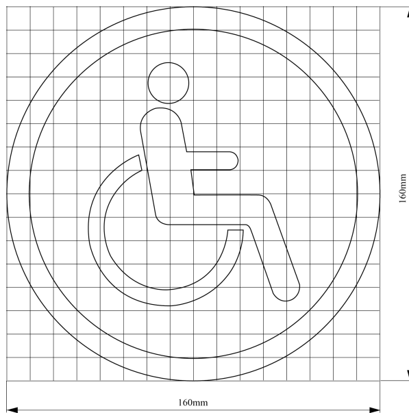
方格尺寸图
